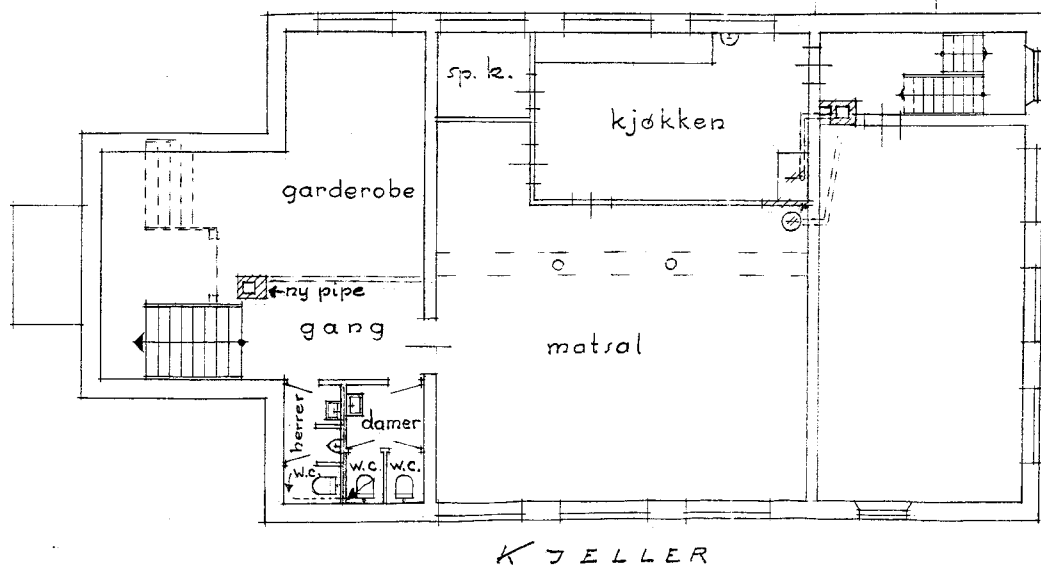
Tegning for ombyggingen i 1953.
